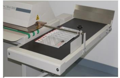
100冊(1/4"で綴じた場合)まで排紙できる 500mm 幅のコンベヤ・・・オプション
