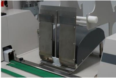
長さ 76~250mm までの成形済みハンガーの自動フィーダー (100本まで)・・・オプション
